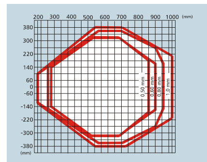
Modèle longue distance (DS4600A-2100)
