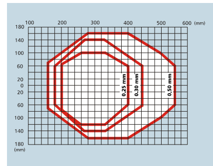
Modèle moyenne distance (DS4600A-2000)
