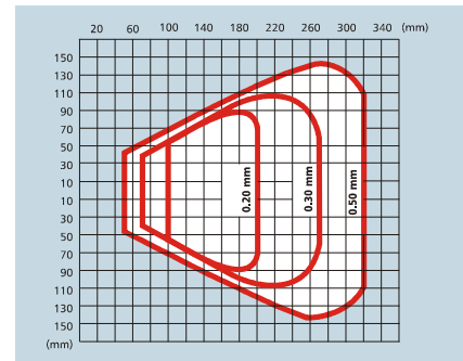
Modèle haute densité (DS4600A-2200)
